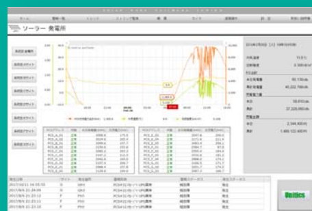
開発画面例
