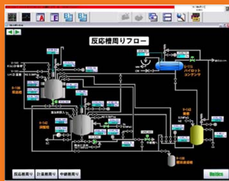
開発画面例
