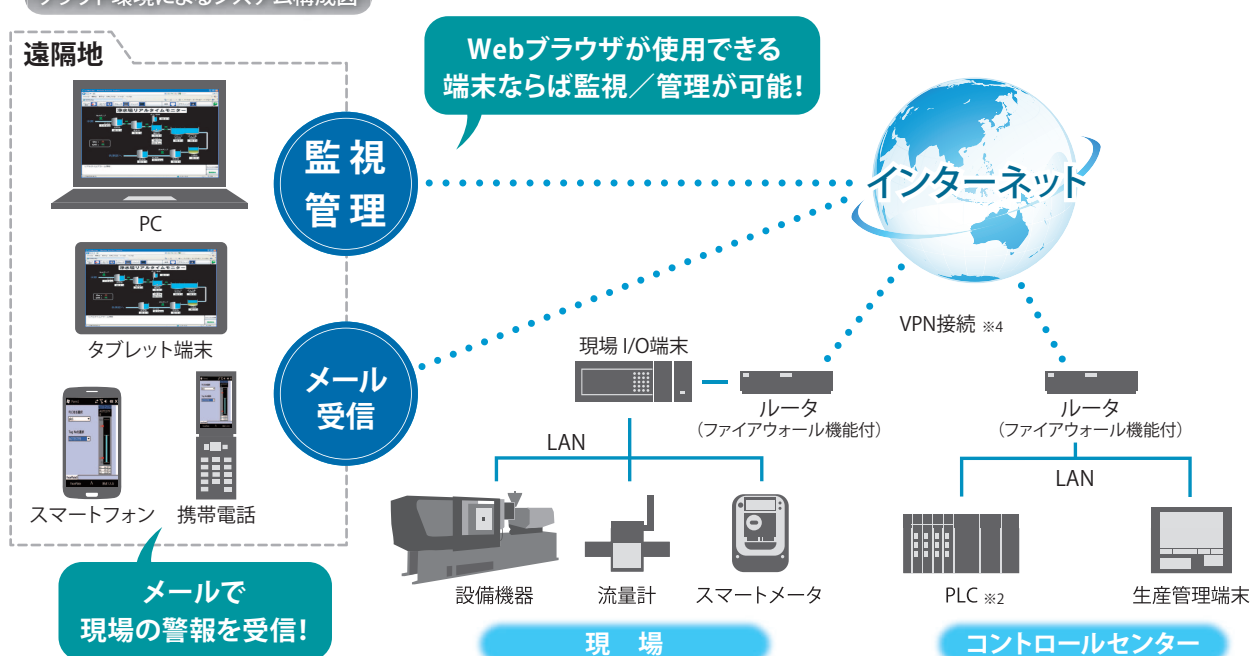
クラウド環境によるシステム構成図
